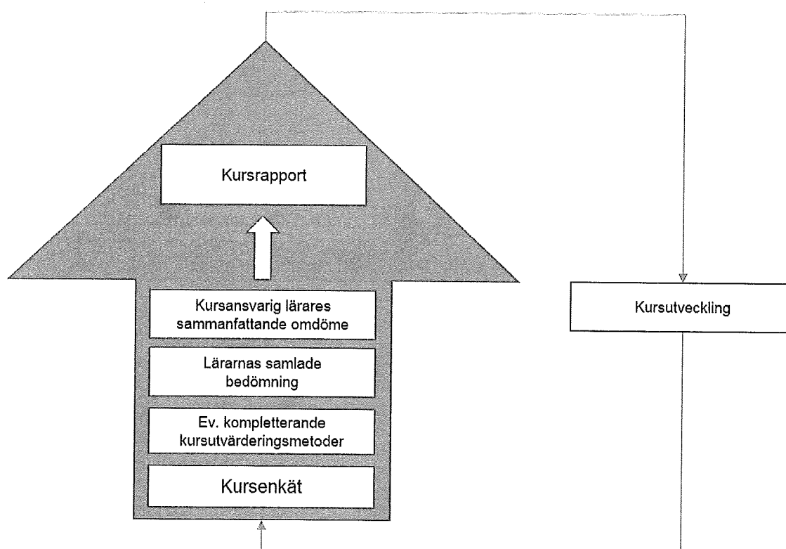
Figur 1: Kursutvärderingsprocessens huvudkomponenter
